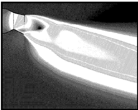
Fig. 1.- CFD Model of a TVN
