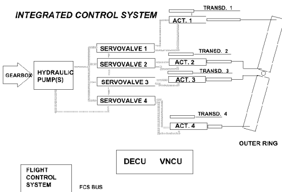
Fig. 16.- TVN Control System
