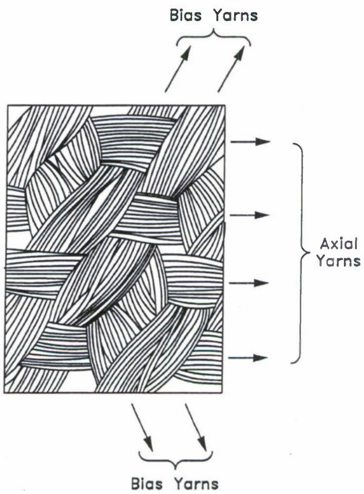
FIG. 17
