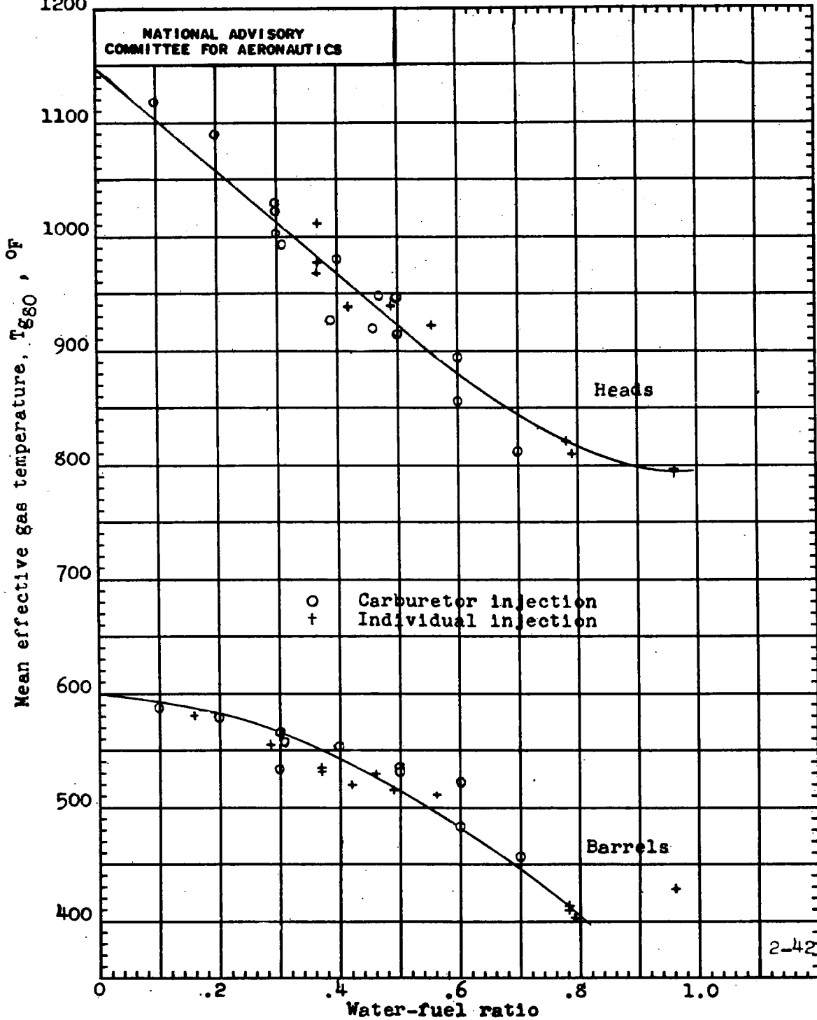
(b) Fuel-air ratio, 0.05.
