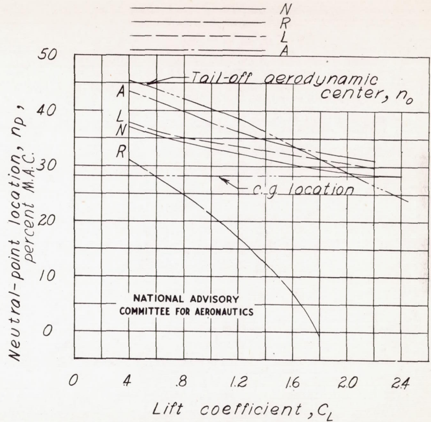
(d) \delta_f = 37^\circ ; power on.
