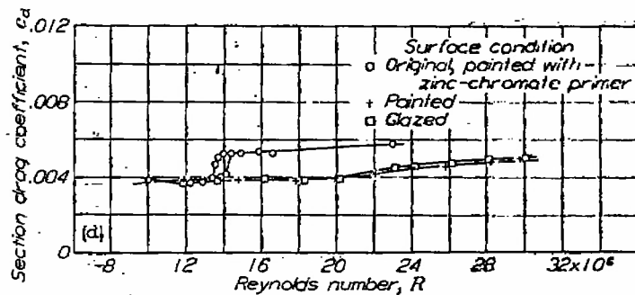
(d) Model 4, NACA 66(215)-116 \left\{ \begin{matrix} \alpha=1.0, c_l=0.2 \\ \alpha=0.6, c_l=-0.1 \end{matrix} \right\} airfoil section. c_l=0.1 .
