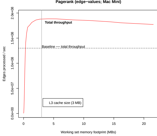
(a) Mac Mini: Pagerank / edge values
