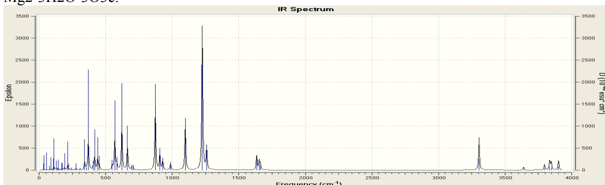
Mg2-3H2O-3O3c:
