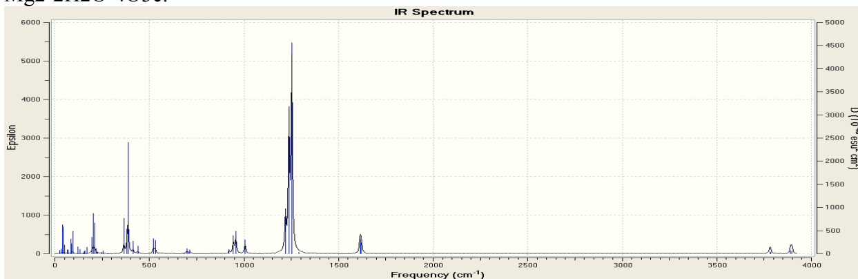
Mg2-1H2O-5O3c:
