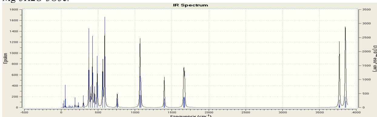
Mg-3H2O-3O3c:
