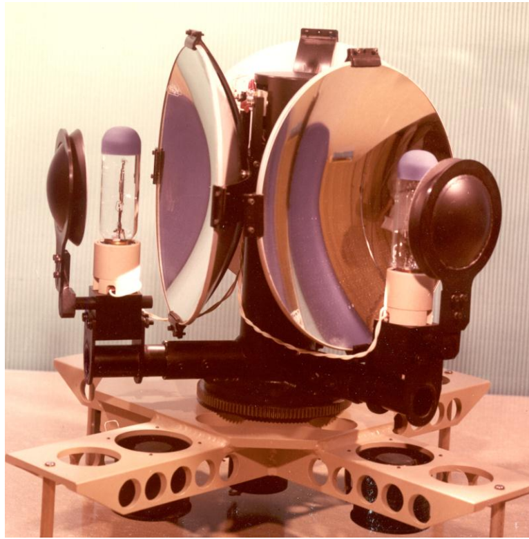
IR Beacon
