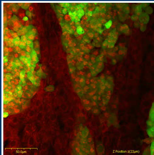
OB + BC
