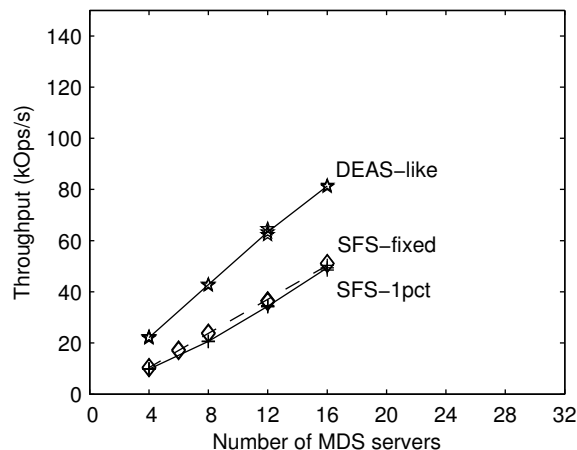
(d) Small constellation NFS throughput
