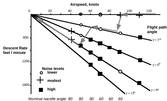
Fig. 3. Noise abatement strategy.
