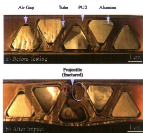
Figuur 21 Resultaat van een impacttest op configuratie (d) uit figuur 20 met een bolvormig RVS-projectiel met een diameter van 12 mm en een snelheid van 613 m/s [35].
