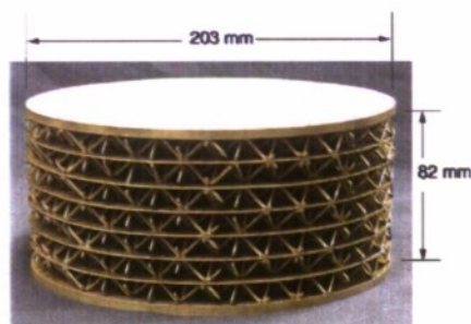
Figuur 19 Voorbeeld van een RVS sandwichconstructie voor het opvangen van onderwaterschokbelasting [34].
