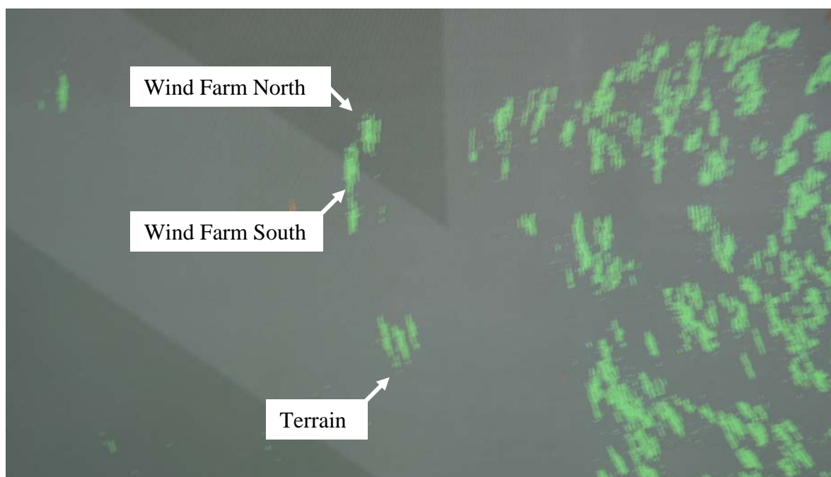
Figure 1 - Background Video.
