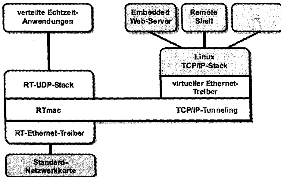
Abbildung 3.13: Der Aufbau von RTnet [9]
