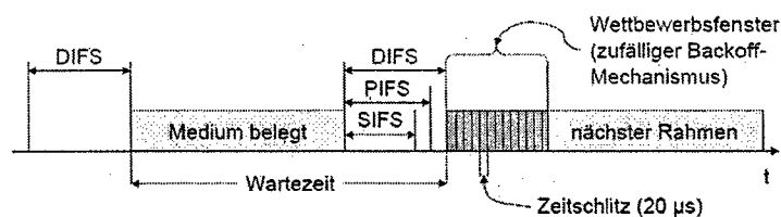
Abbildung 3.10: Die unterschiedlichen IFS bei MACA [7]
