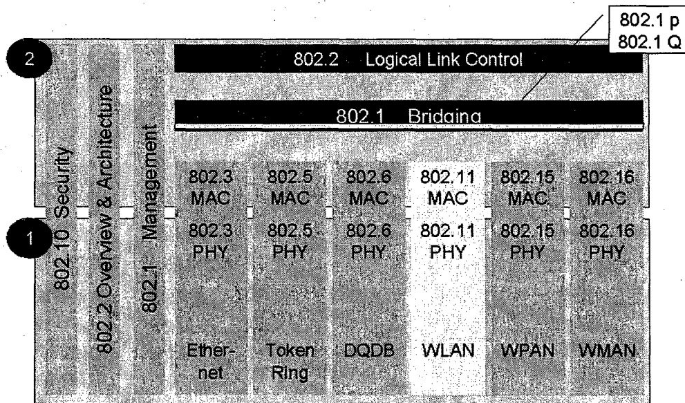
Abbildung 5.3: Einordnung von WLAN nach 802.11
