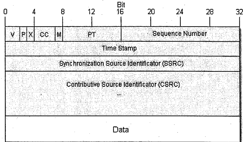
Abbildung 3.12: Der RTP Frame [12]
