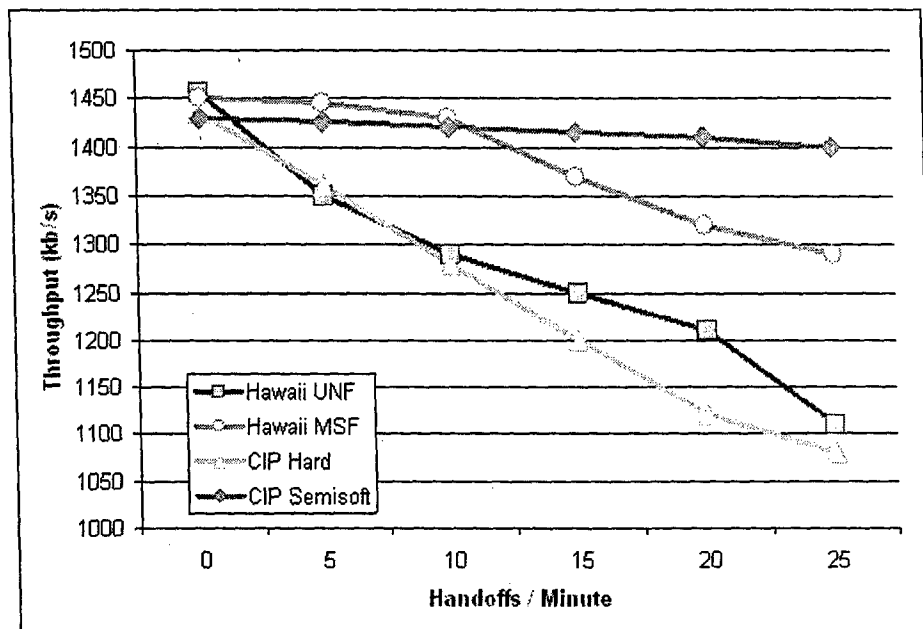
Abbildung 4.12: TCP Durchsatz auf Anwendungsschicht, aus [8]
