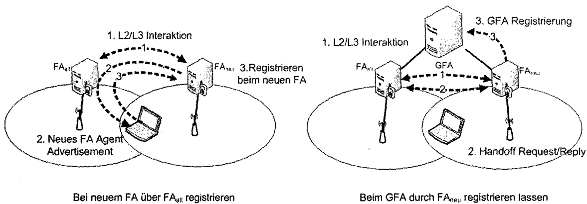
Abbildung 4.6: Handoff Mechanismen für a) Fast Handoff und a) Proactive Handoff [4].
