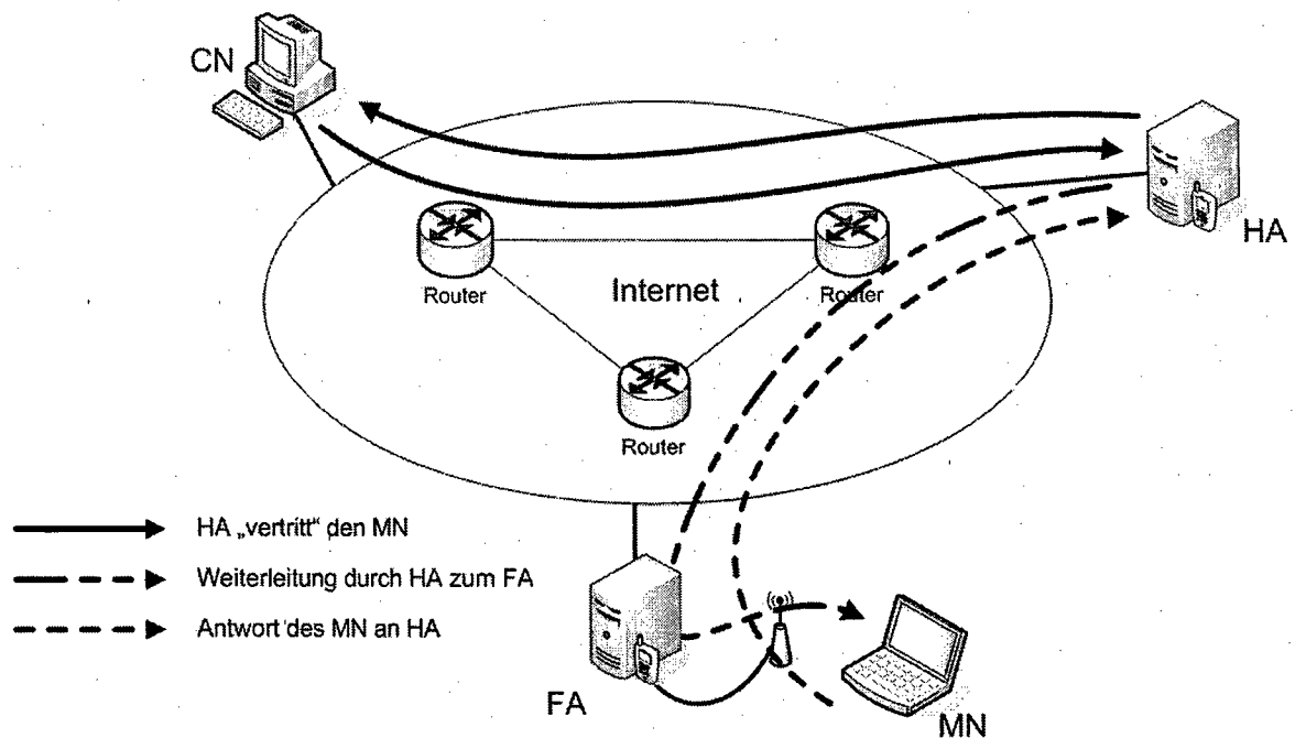
Abbildung 4.1: Mobile IP mit Reverse Tunneling
