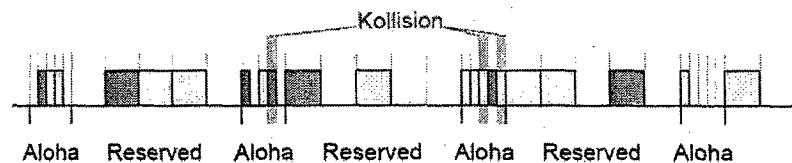
Abbildung 3.8: DAMA mit Slotted Aloha zur Reservierung [7]
