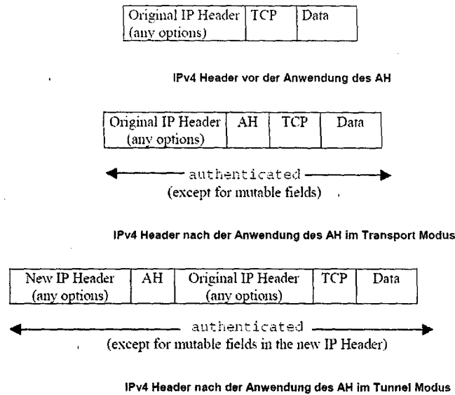
Abbildung 2.11: Das Authentication-Header-Protokoll(AH)[28]
