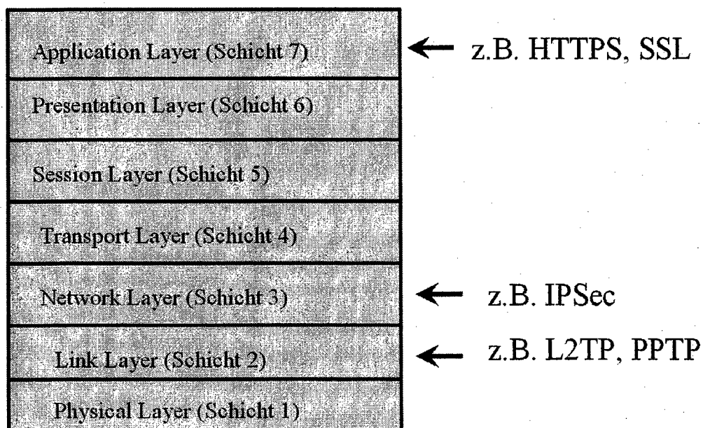
Abbildung 2.10: OSI-Schichten
