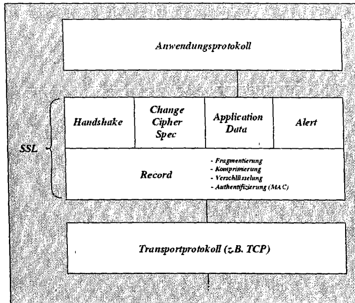
Abbildung 2.14: Das SSL-Schichtenmodell[23]
