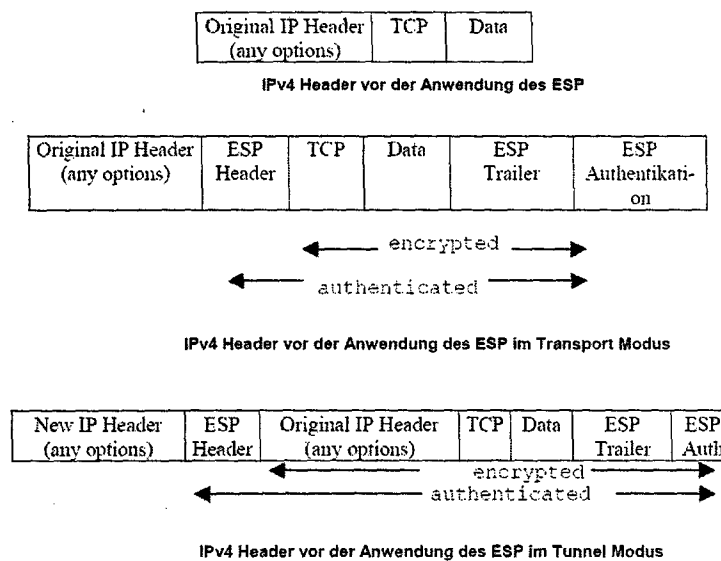
Abbildung 2.12: Das Encapsulating-Security-Payload-Protokoll(ESP)[28]
