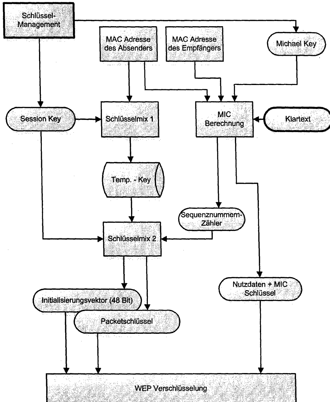
Abbildung 6.4: TKIP – Verschlüsselung
