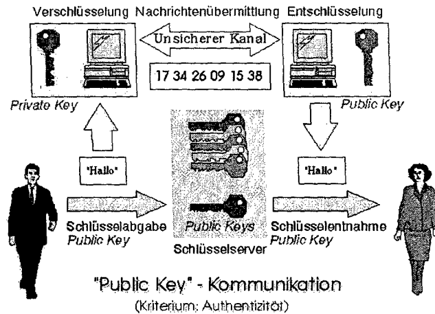
Abbildung 2.9: Asymmetrische Verschlüsselung[12]
