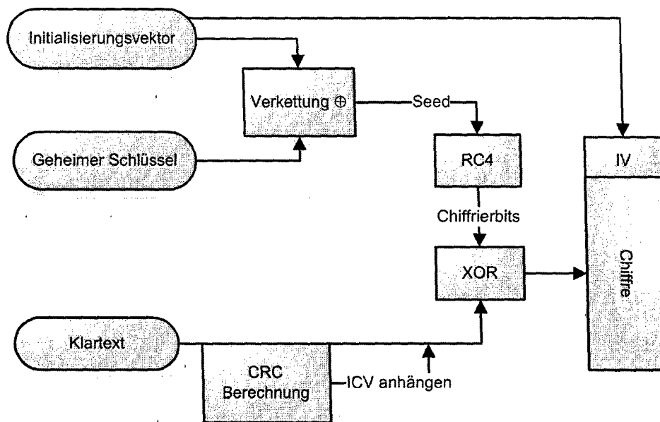
Abbildung 6.1: WEP – Verschlüsselung
