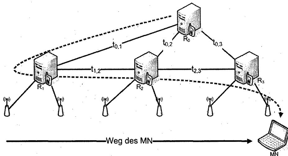
Abbildung 4.11: Eine suboptimale Route nach mehreren Handoffs
