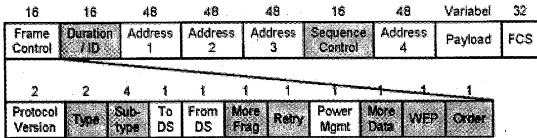
Abbildung 5.5: MAC-Frame nach IEEE 802.11
