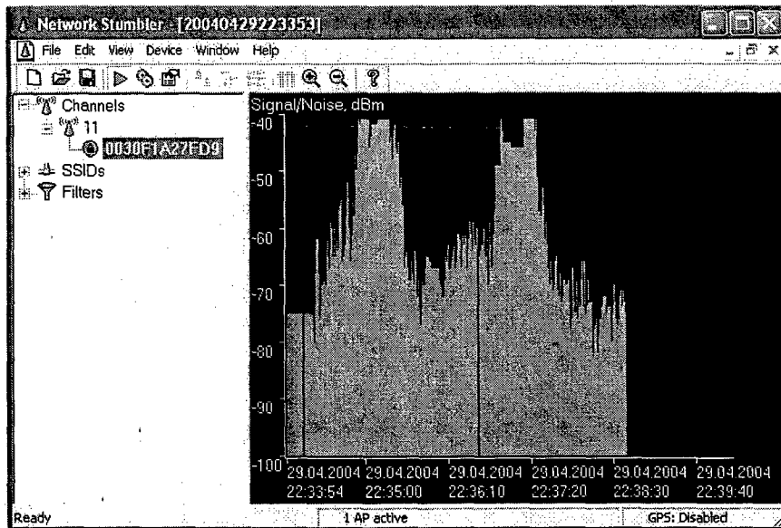
Abbildung 1.5: Netstumbler: Modus-Sendeleistung [23]
