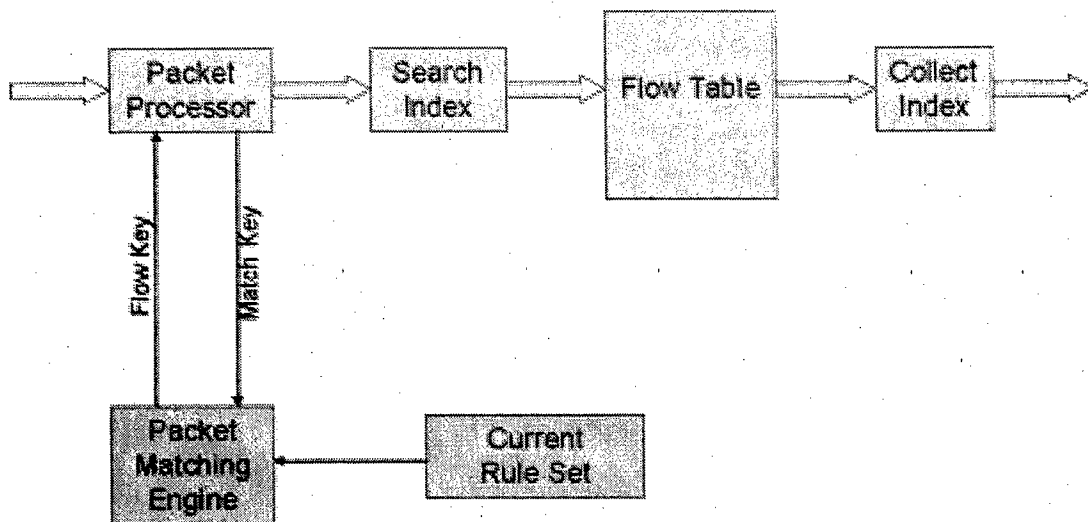
Abbildung 5.2: Paketverarbeitung nach RTFM
