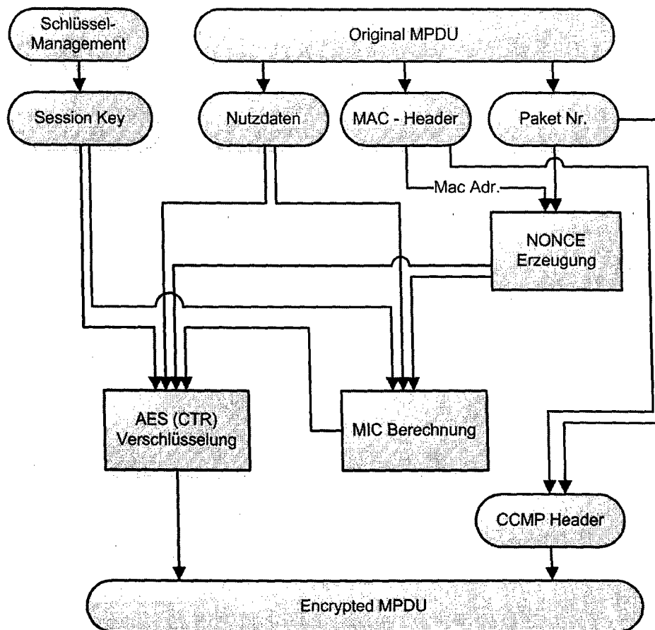
Abbildung 6.7: CCMP – Verschlüsselung
