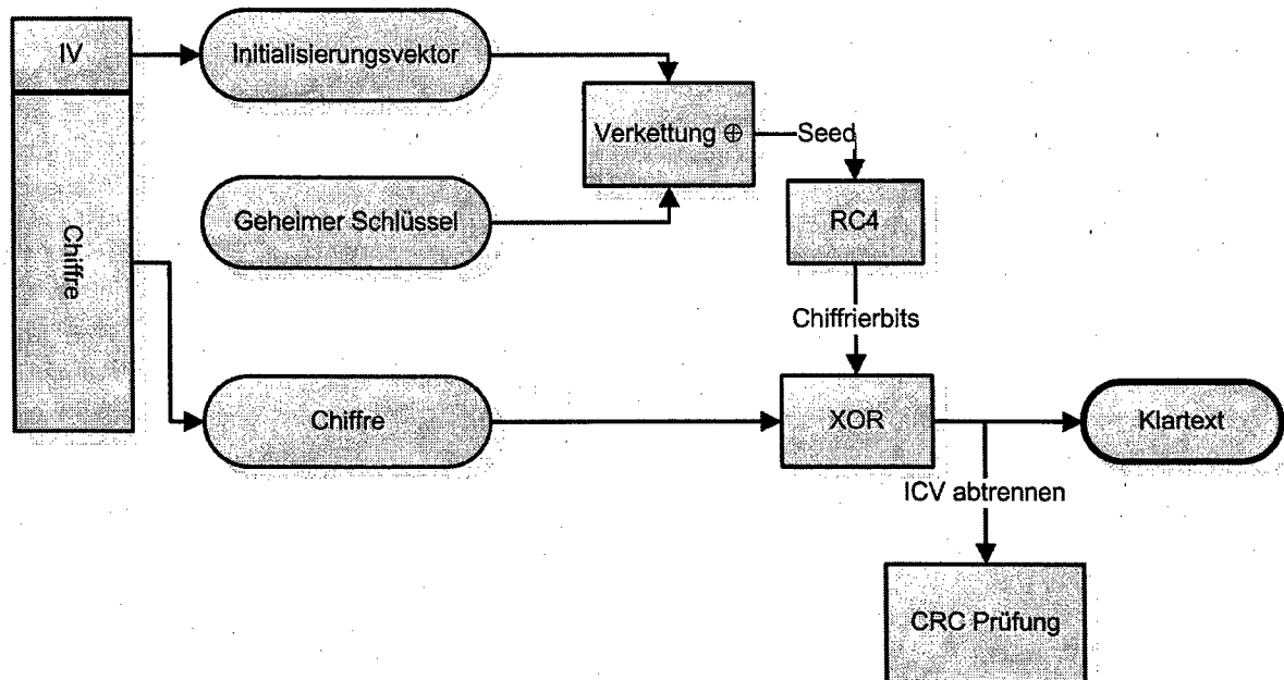
Abbildung 6.2: WEP – Entschlüsselung
