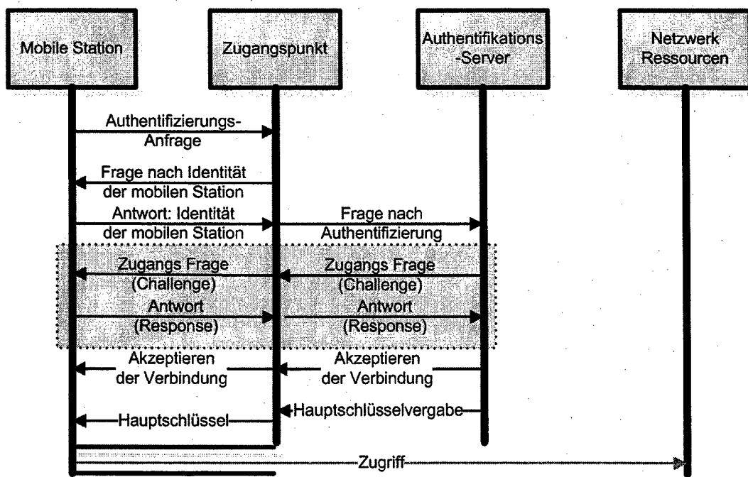
Abbildung 6.10: 802.1x Authentifizierung
