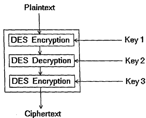
Abbildung 2.8: Triple-DES Verschlüsselung[12]
