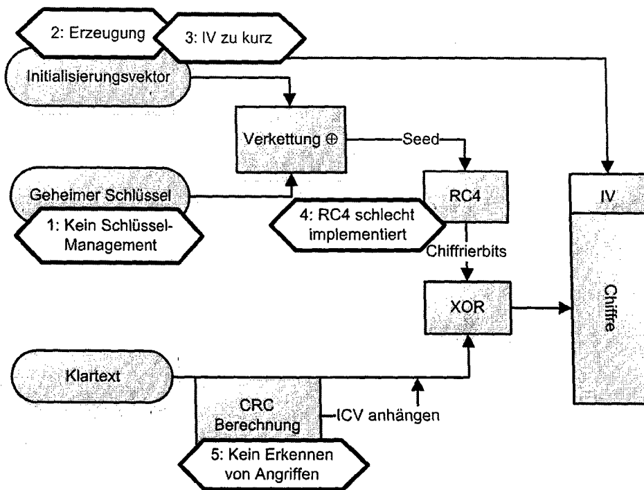
Abbildung 6.3: WEP – Schwachstellen
