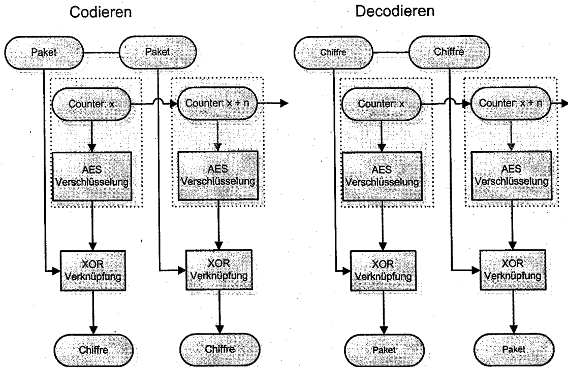
Abbildung 6.6: AES – Counter
