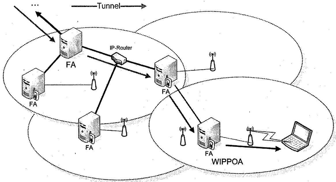
Abbildung 4.4: Das Prinzip von Hierarchical Tunneling
