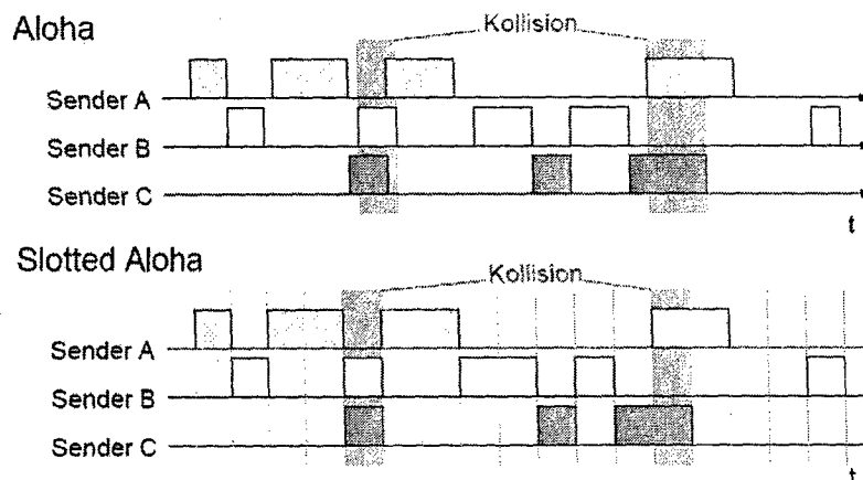
Abbildung 3.7: Schema von Aloha, bzw. Slotted Aloha [7]
