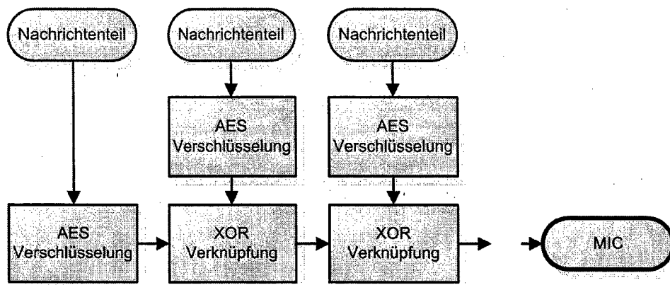
Abbildung 6.8: CCMP – MIC Berechnung
