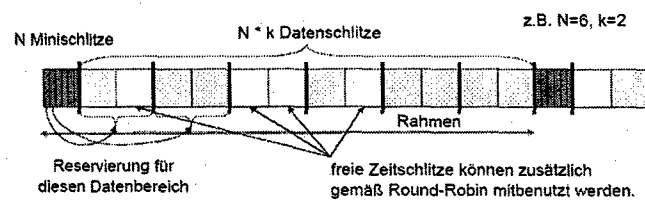
Abbildung 3.9: DAMA mit implizierter Reservierung [7]
