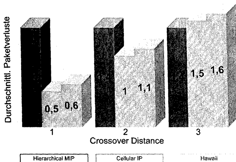
Abbildung 4.10: UDP Paketverluste während des Handoffs, entnommen aus [8]
