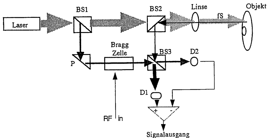
Fig. 5. Prinzipieller optischer Aufbau eines Laser-Doppler-Vibrometers. 24
