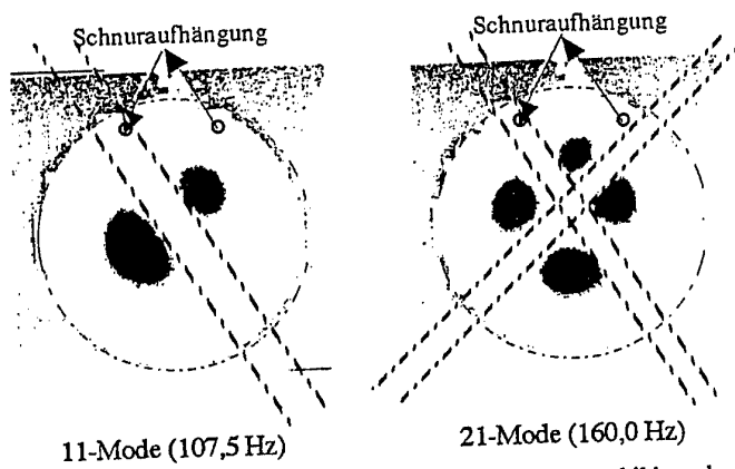
Fig. 30. Lage der Knotenmeridiane (gestrichelte Linien) in zwei PSV-Schwingungsbildern der 11-Mode und 21-Mode bei fengluo AV.87 in Konkordanz mit den Aufhängelöchern und der Schnuraufhängung (Pfeile). 11
