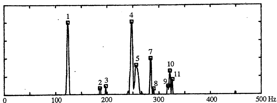
Fig. 39. Spektrum agung (MIM 61-11) starker Anschlag, Bandbreite 0 - 500 Hz.
