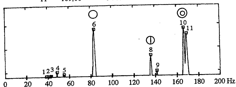
Fig. 54. Spektrum gong suwukan (AV.88) mittelstarker Anschlag; Modenzuordnung (nach Twork); Bandbreite 0 - 200 Hz.
