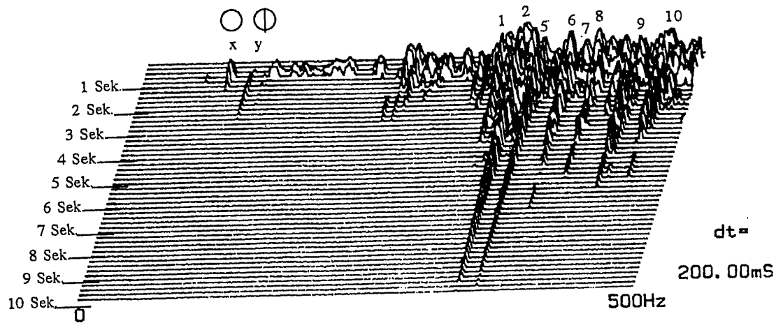
Fig. 29. Wasserfalldiagramm fengluo (AV.87) starker Anschlag mit Zuordnung zweier Eigenschwingungen (01, 11) aus der PSV-Analyse (nach Twork); Bandbreite 0 - 500 Hz.
