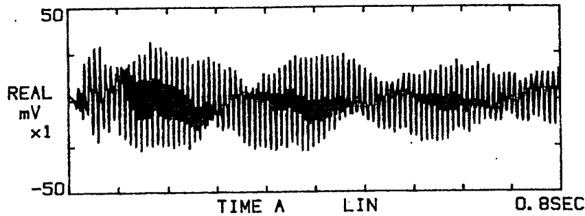
Fig. 11. Schwabungen eines balinesischen kempur (CB.95) mit ca. fünf Schlägen pro Sekunde (FFT-Analyse mit I. Teilton bei 113,75 Hz, das etwa dem Ton b -42 \mu entspricht).
