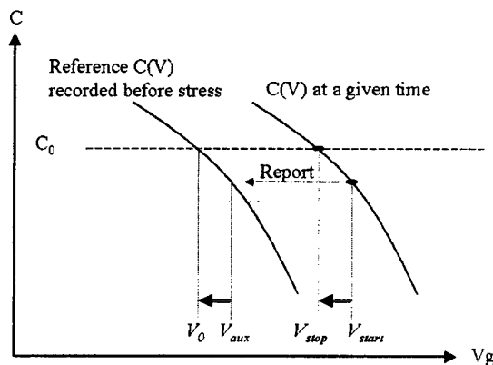
Fig. 2 : Voltage correction
