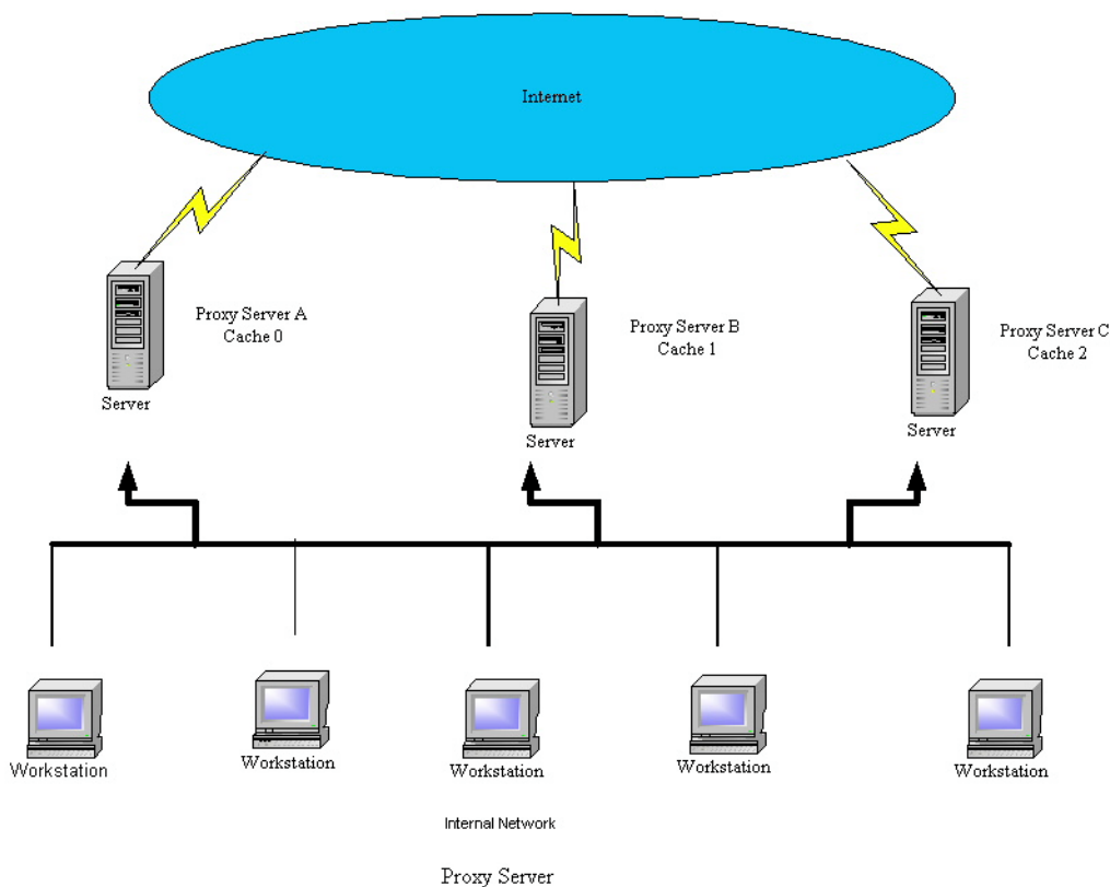
Fig. 1. Proxy servers
