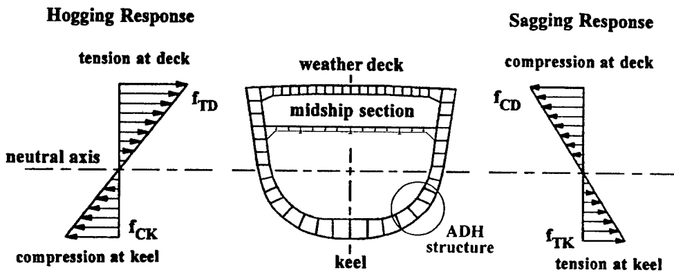
Actual Longitudinal Primary Bending Stresses
