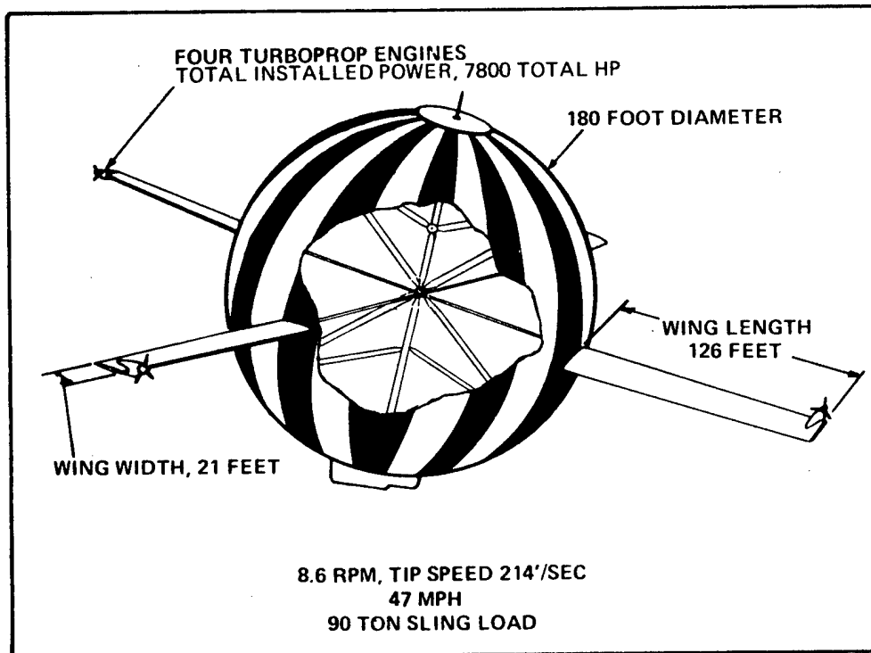
90 Ton Aerocrane
