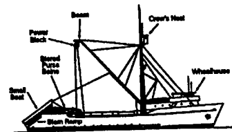
Purse Seiner
