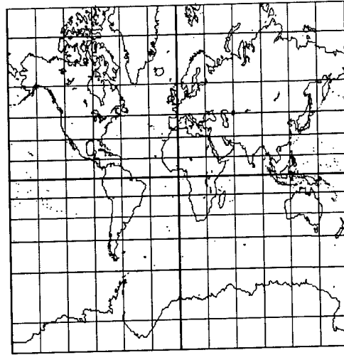
MERCATOR
