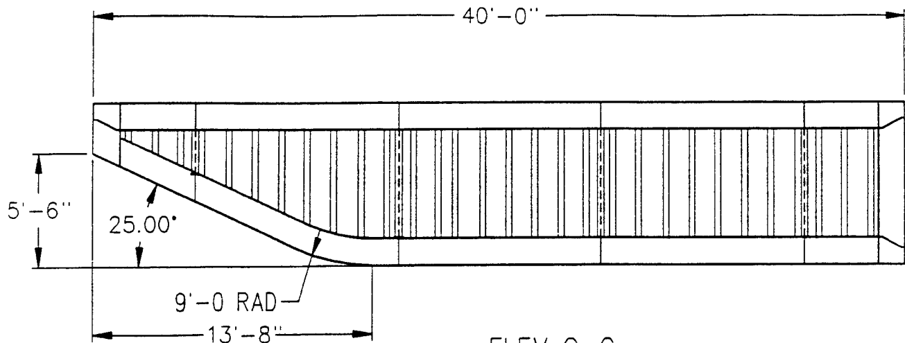
ELEV G-G
