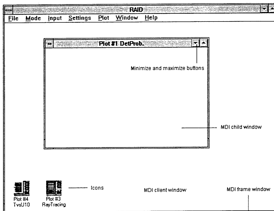
Figuur 4.5: MDI Applicatie
