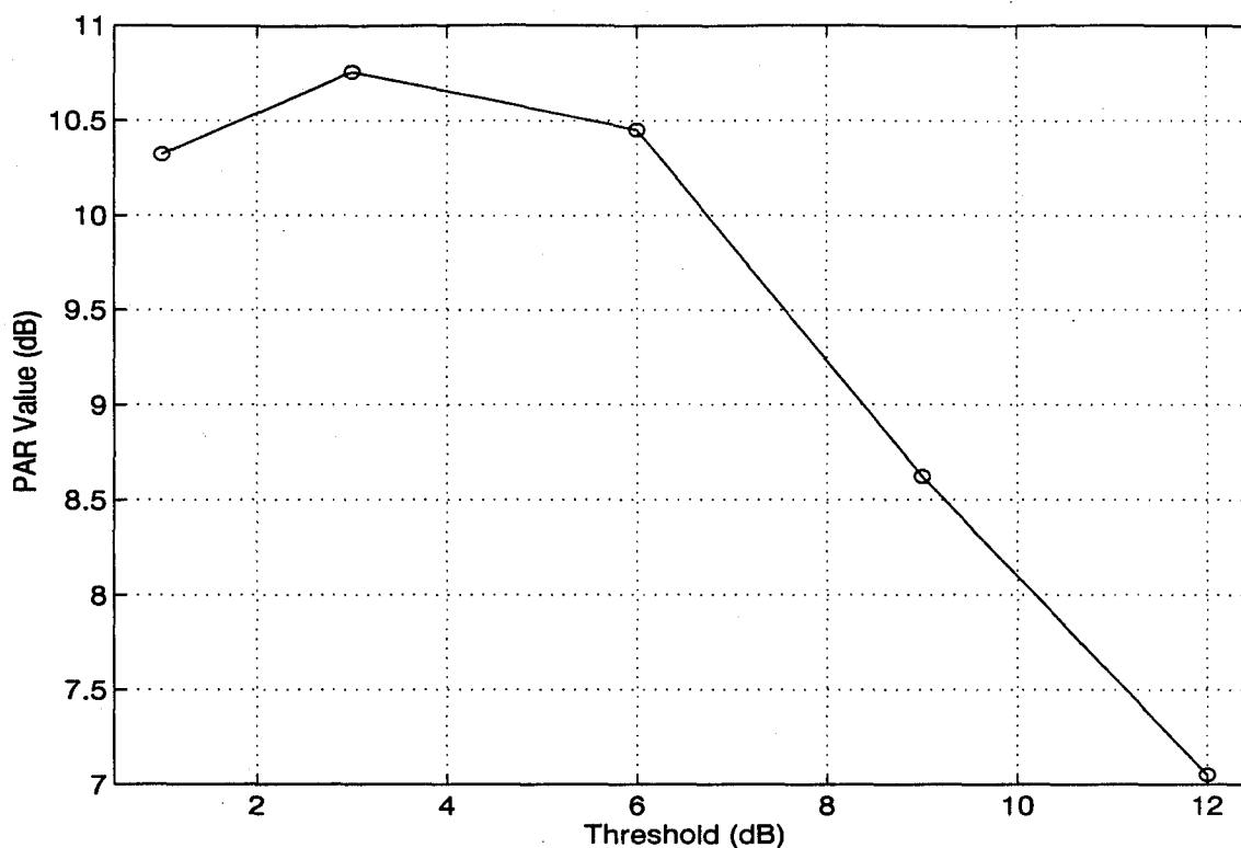
Figure 25. PAR Curve for Scenario #4
