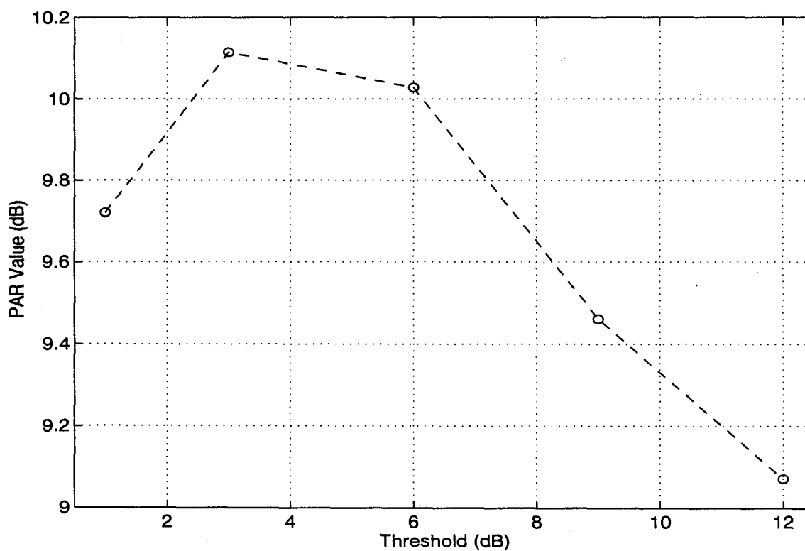
Figure 27. PAR Curve for Scenario #8
