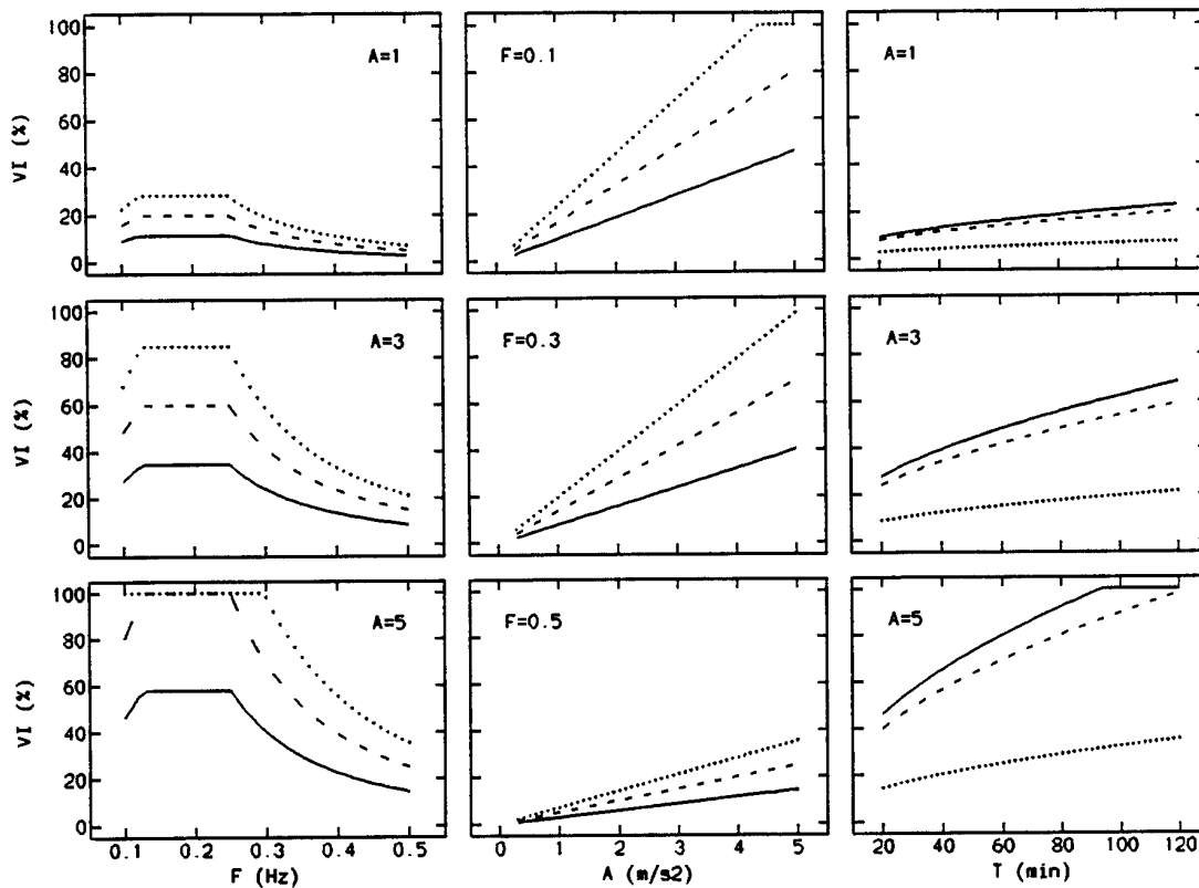
Fig. 4 VI versus frequentie (F), amplitude (A) en tijd (T). Hele lijnen representeren T=20 min dan wel F=0.1 Hz, onderbroken lijnen T=60 min of F=0.3 Hz en stippellijnen T=120 min of F=0.5 Hz.
