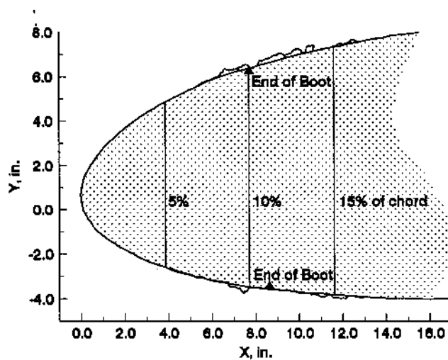
a). Flap = 0°
