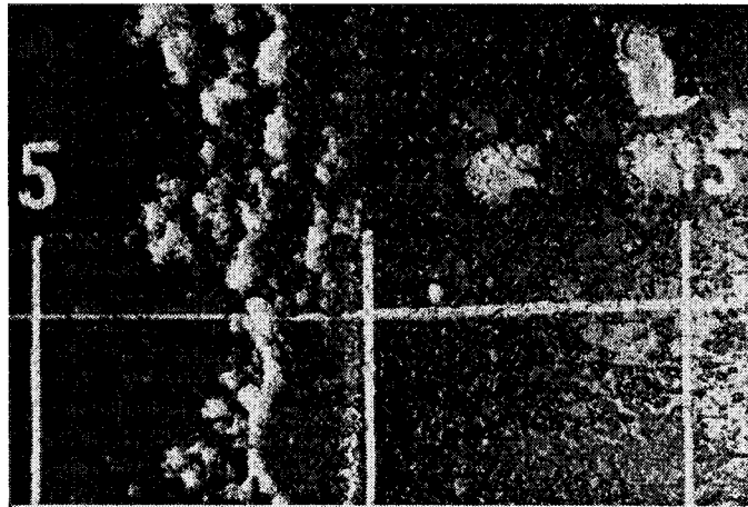
a). Run 3, T_t = 32^\circ\text{F} , V = 125 mph
