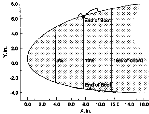
a). Run 43a, STA 36 tracing
