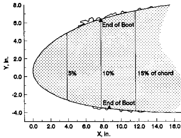
a). Run 43, STA 36 tracing
