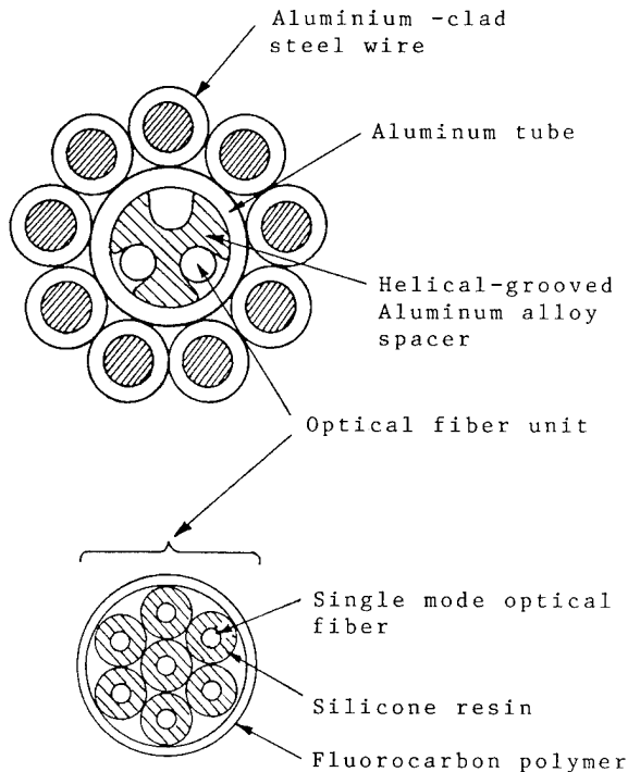
Fig. 8 Structure of OPGW
