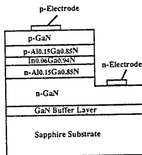
Fig.1 InGaN/AlGaN DH LEDs.
