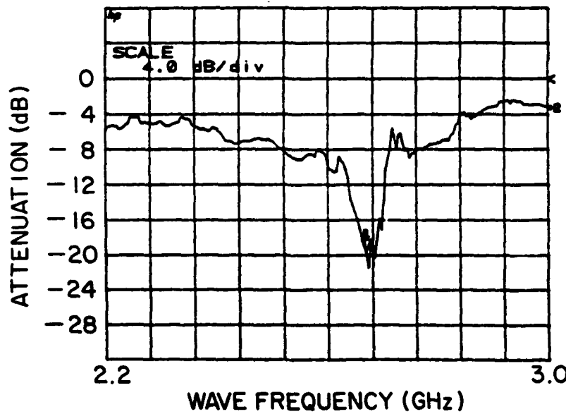
Fig.7 Attenuation Vs. frequency for V=700\text{V} ; P=70\text{mTorr} ; B=950\text{Gauss} ; and (a) I=250\text{mA} , (b) I=300\text{mA} .
