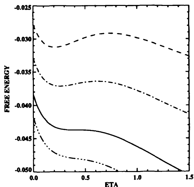
Fig. 4. Free energy \mathcal{F}_v versus \eta at different temperatures: T = 350 (dashed), 380 (dash-dotted), 411 (solid), 430 (dash-dot-dot-dot) K.
