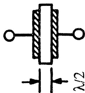
BAW
