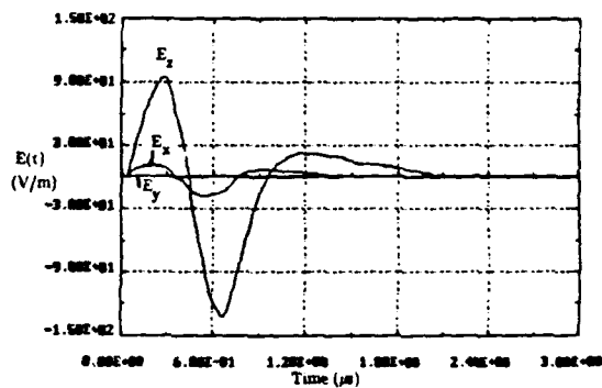
(d) N = 256
