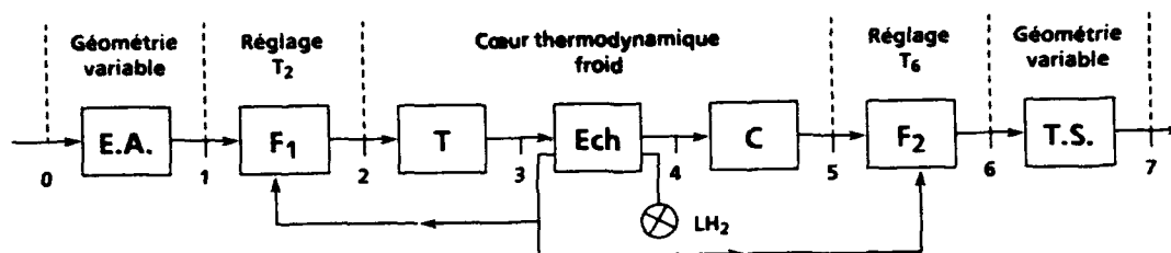
Fig. 1 - Schéma de principe du moteur à composants inversés (Brevet ONERA). Notations : E.A. : entrée d'air - F 1 : foyer 1 - T : turbine - Ech : échangeur C : compresseur - F 2 : foyer 2 - T.S. : tuyère de sortie.
