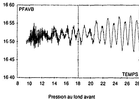
Figure 18 - Calcul du couplage acoustique-émission tourbillonnaire
