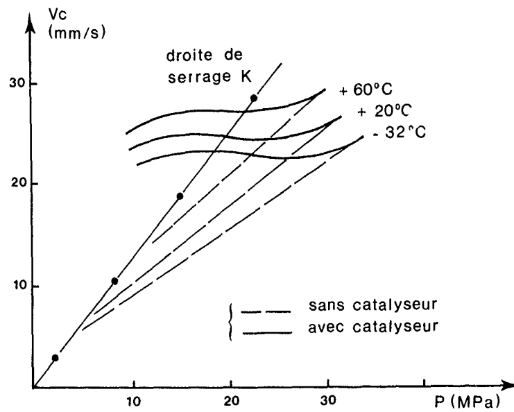
Figure 2: Courbes vitesse-pression typiques d'un propergol double-base
