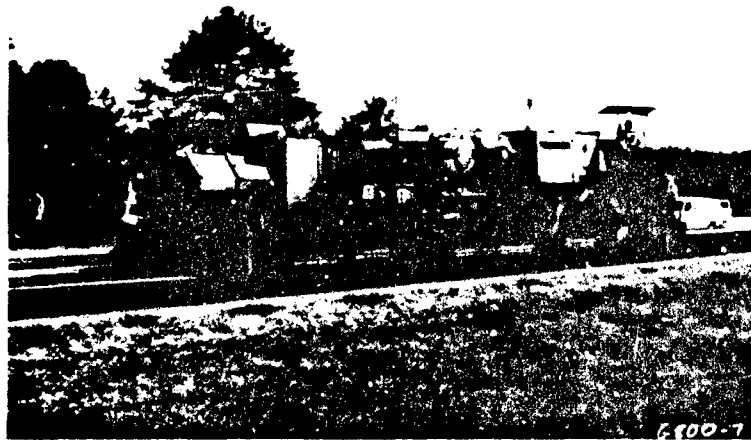
Photo 3. Wirtgen Remixer
