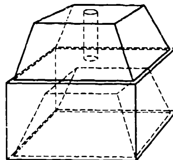
Abb. 16 Kast, Vergleich der Sprengwirkung eines Hohl- und eines Vollkörpers auf eine Eisenplatte. 1911
