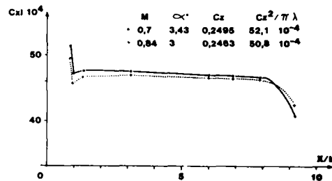
Fig. 21 - Influence de la position du plan aval sur le calcul de la traînée induite. Aile M6 \lambda = 3,8 . Méthode potentielle non conservative 3D. Fluide parfait.
