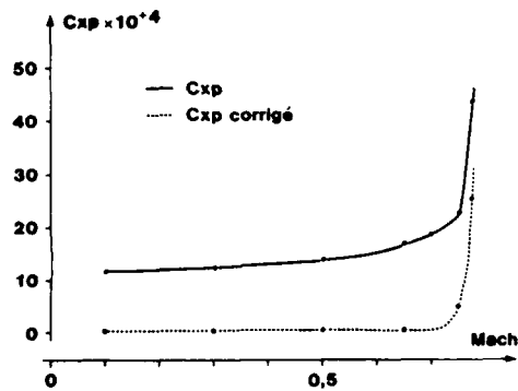
Fig. 7 - Amélioration du calcul du C_x pression Profil NACA0012 C_r = 0 . Fluide parfait Méthodes de calcul potentielles.
