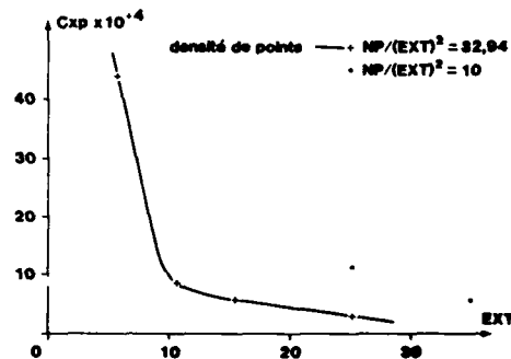
Fig. 3 - Influence de l'extension du maillage Fluide parfait 2D. Profil NACA0012 M = 0,1 \alpha = 0 .
