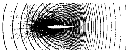
Fig. 15 - Schéma du maillage. Méthode potentielle différences finies 3D.
