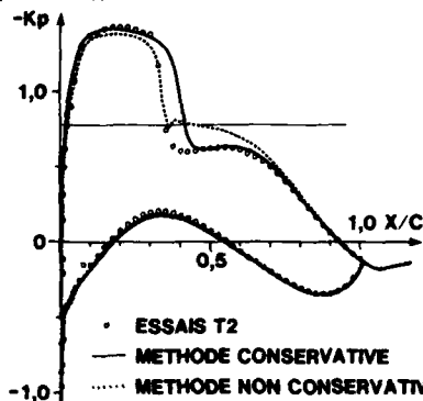
Fig. 11 - Prédiction des répartitions de pression. Profil CAST 7 M = 0,7 \alpha = 2^\circ . Méthodes potentielles couplées (couplage fort). T.D. R_e = 4,5 \cdot 10^6 .
