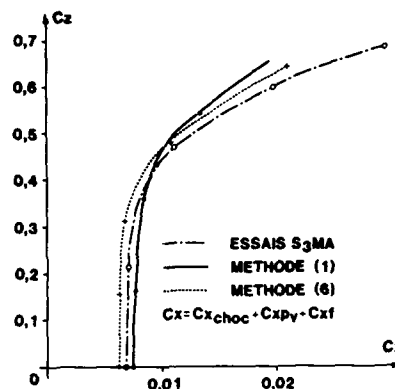
Fig. 9 - Prédiction de la traînée. Profil NACA0012 M = 0,7 Re = 3,6 \cdot 10^6 . Méthodes potentielles couplées (couplage faible). T.N.
