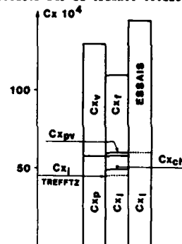
Fig. 25 - Prédiction de la traînée. Aile M6 \lambda = 3,8 M = 0,7 C_x = 0,245 Re = 7,3 \cdot 10^6 T.N. Méthode potentielle couplée 3D.
