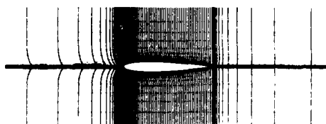
Fig. 16 - Schéma du maillage. Méthode potentielle éléments finis 3D.
