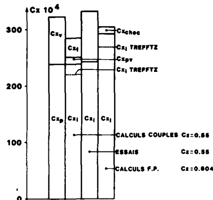
Fig. 27 - Prédiction de la traînée. Aile non symétrique \lambda = 4 M = 0,8 C_x = 0,55 R_e = 3,7 \cdot 10^6 T.D. Méthode potentielle couplée 3D.
