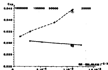
Fig. 14 - Influence du nombre de points de maillage sur le C_{xp} . Fluide parfait 3D. Méthodes potentielles. Cas transsonique.
