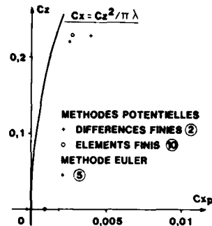
Fig. 19 - Prédiction de la traînée de pression. Fluide parfait 3D. Aile elliptique M = 0,6 \lambda = 10,2 .
