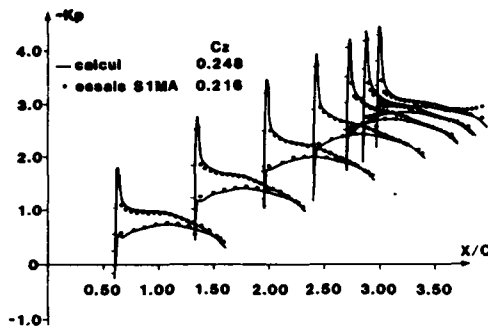
Fig. 26 - Répartitions des pressions. Aile M6 \lambda = 3,8 M = 0,7 C_x = 0,245 R_e = 7,3 \cdot 10^6 T.M.
