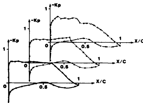
Fig. 28 - Répartition des pressions. Aile non symétrique \lambda = 4 M = 0,8 C_x = 0,55 R_e = 3,7 \cdot 10^6 T.D.
