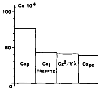
Fig. 20 - Prédiction de la traînée de pression. Aile elliptique M = 0,1 \lambda = 21 \alpha = 5^\circ . Méthode potentielle non conservative 3D. Fluide parfait.
