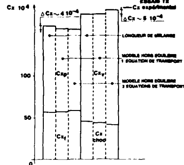
Fig. 12 - Prédiction de la trainée. Influence du modèle de turbulence. Méthode potentielle conservatrice (couplage fort). Profil CAST 7 M = 0,7 \alpha = 2^\circ R_e = 4,5 \cdot 10^6 .
