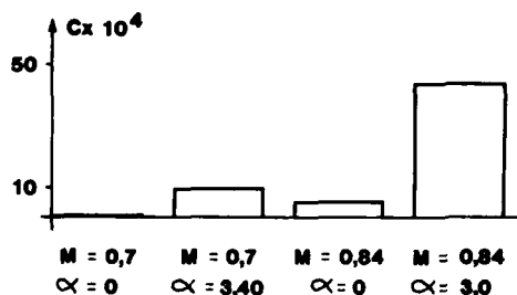
Fig. 24 - Prédiction de la traînée de choc Aile M6 Méthode potentielle non conservative 3D.
