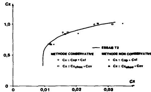
Fig. 10 - Prédiction de la trainée. Profil CAST 7 M = 0,7 R_e = 4,5 \cdot 10^6 . Méthodes potentielles couplées (couplage fort). T.D.
