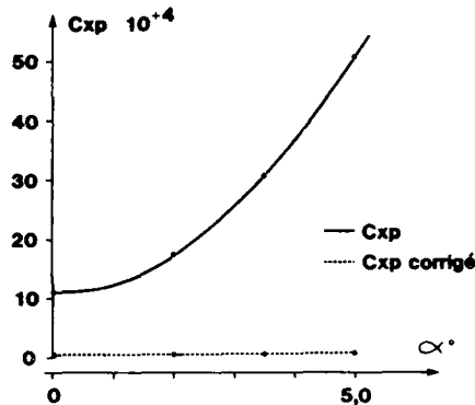
Fig. 6 - Amélioration du calcul du C_x pression Profil NACA0012 M = 0,1 . Fluide parfait Méthodes de calcul potentielles.
