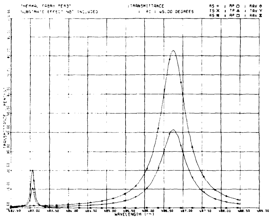
(d) Angle of incidence 45^\circ
