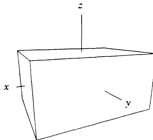
n=\infty
