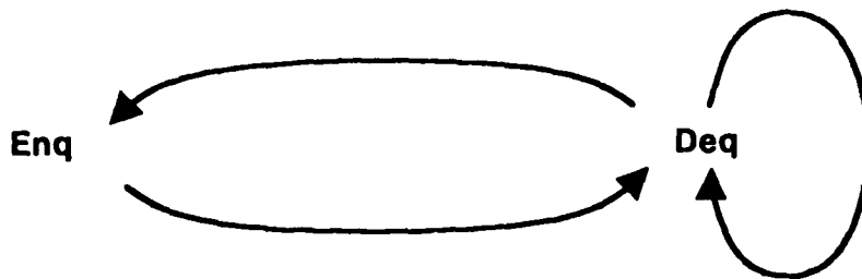
Fig. 9. An Atomic FIFO Queue
