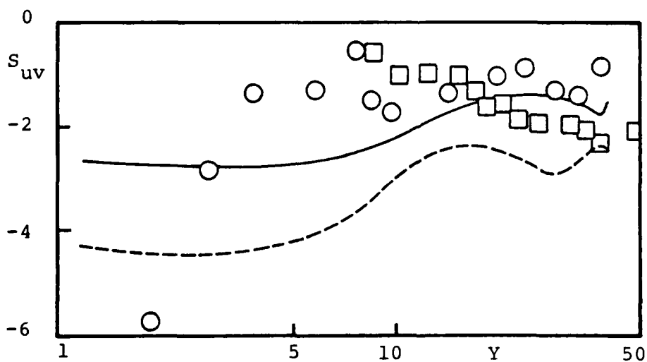
b. Skewness
