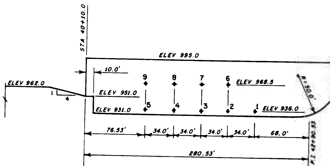
ELEVATION
