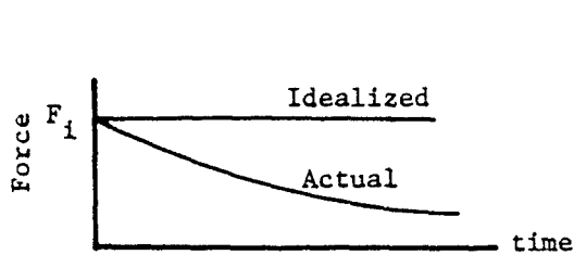
Fig. 1 Force Function
