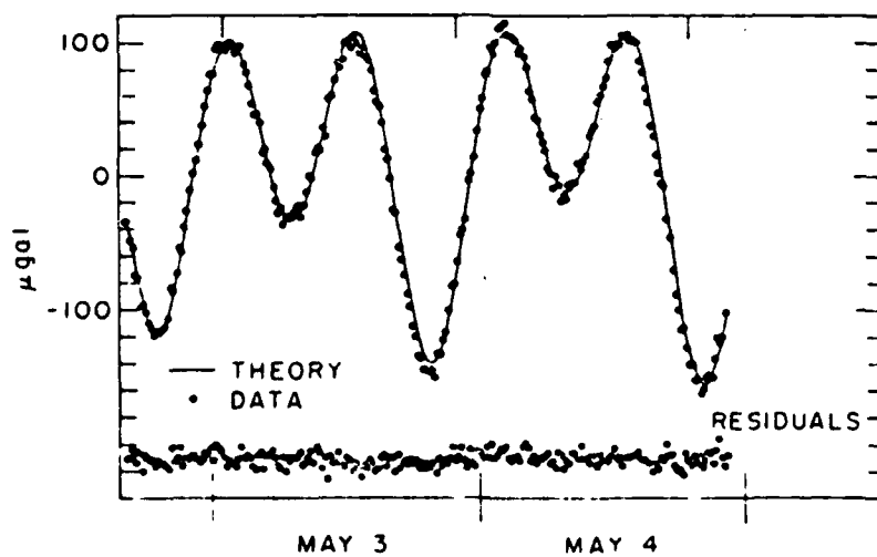
Fig. 7. Gravity tide.
