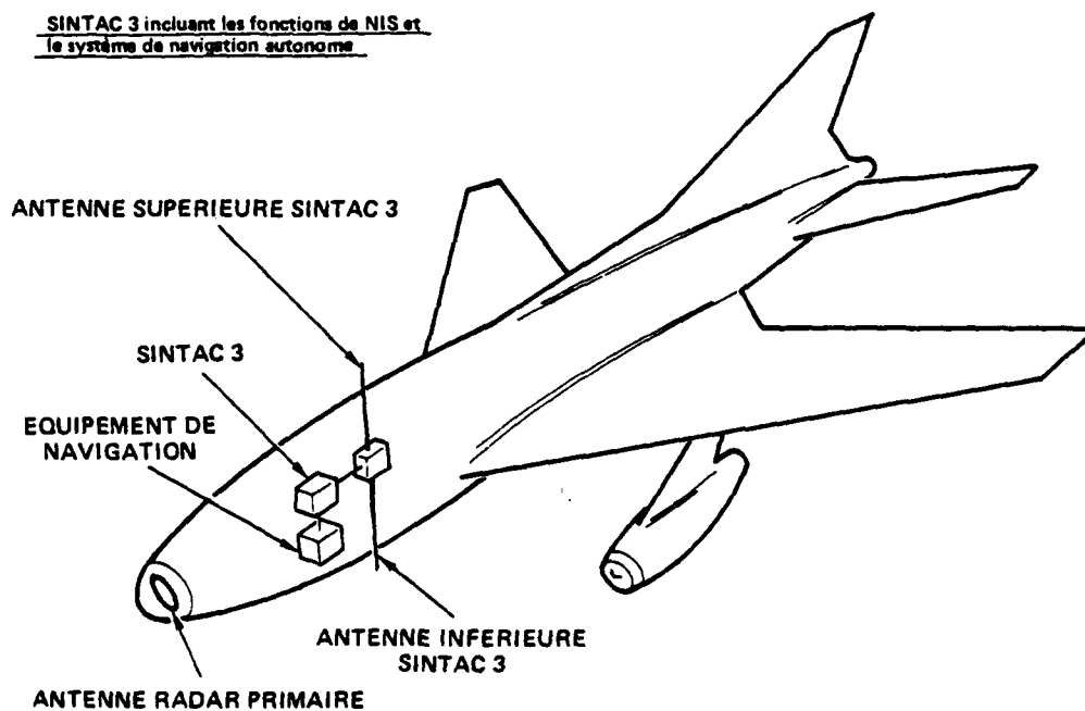
Fig.3(b) Equipements avions du MIDS et du NIS
