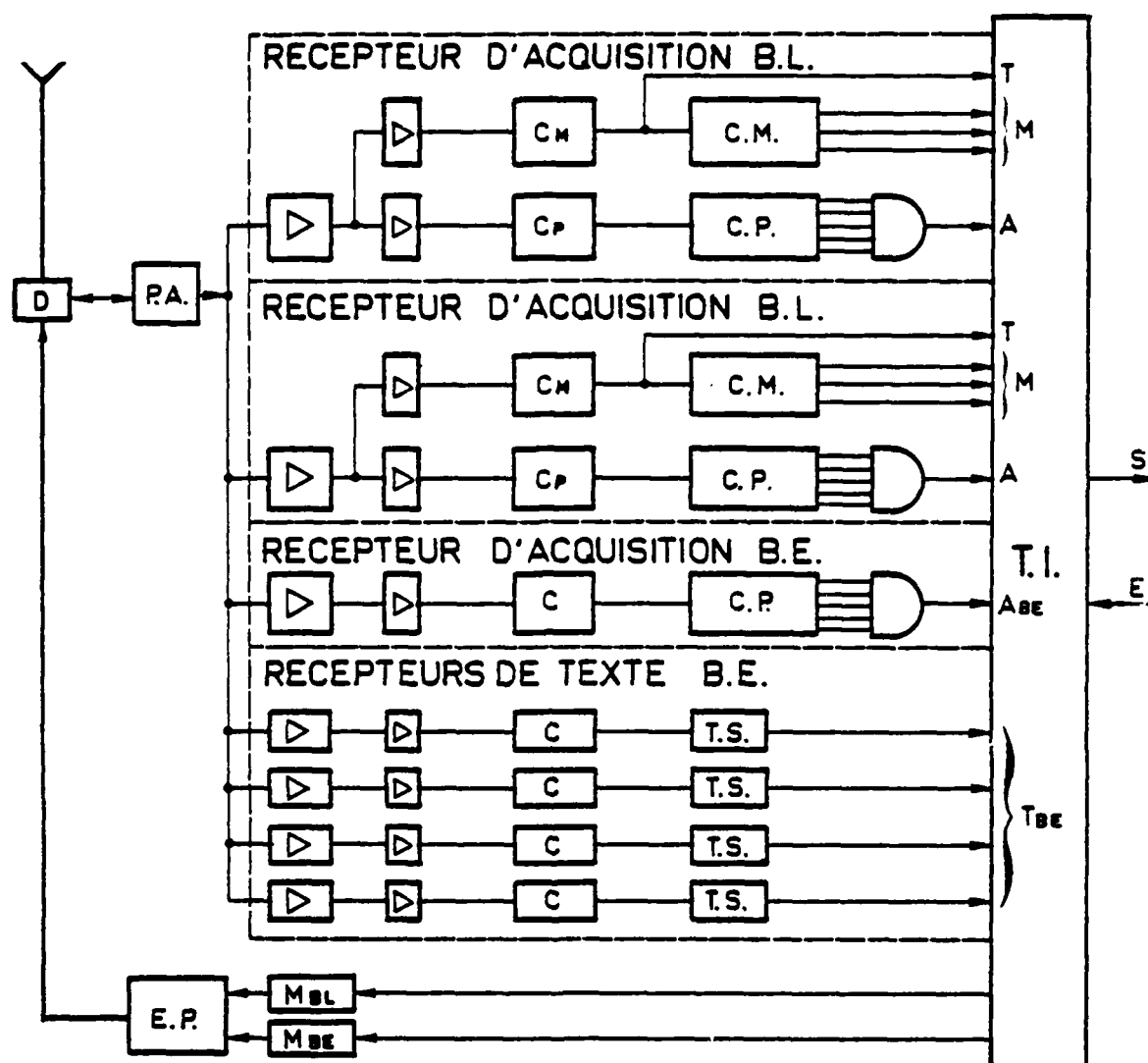
Fig.8 Terminal A2
