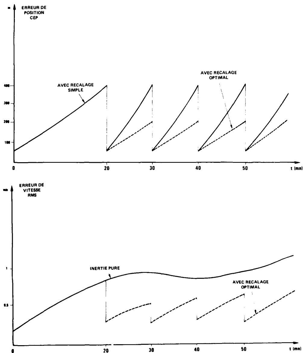
Figure 5 : PERFORMANCE DU FILTRE OPTIMAL DANS LE CAS D'UNE MISSION TYPE DE PÉNÉTRATION ET D'ATTAQUE AU SOL INERTIE - CORRÉLATION D'ALTITUDE
