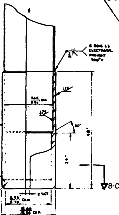
DETAIL 10-A
