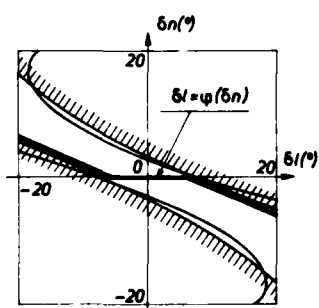
Fig. 9 — Avion A : Surface de bifurcation. Loi de pilotage \delta l = \varphi(\delta n) .
