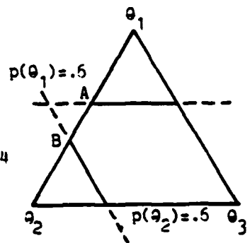
Fig. 2.3c Incoherence
