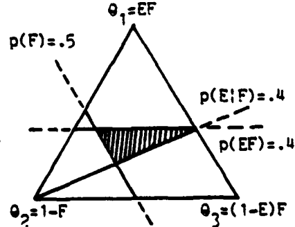
Fig. 2.4b Incoherence
