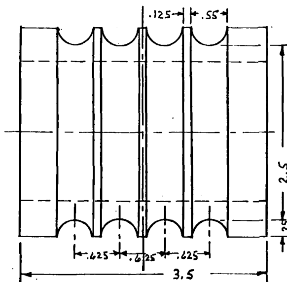
Four-Groove Spool
