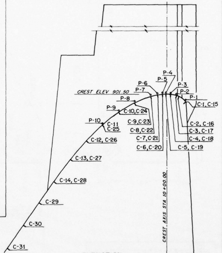
ELEVATION
